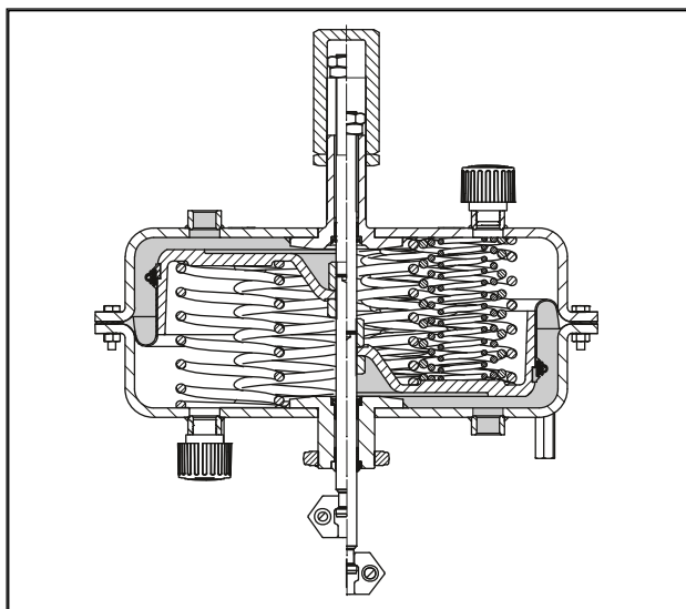
Fig. 3: 1400-60 cm 2 version med mekaniska slaglängdsstopp på båda sidor
