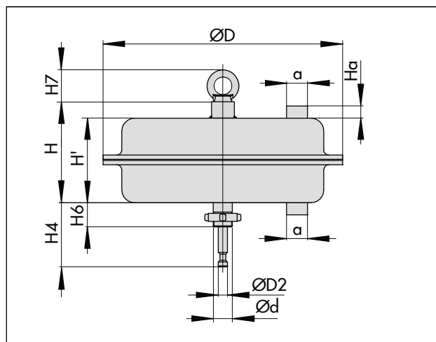
Fig. 4: Typ 3271 med 1400-60 cm 2 ställdonsområde
