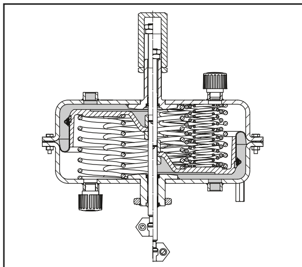
Fig. 3: 1400-60 cm 2 version med mekaniska slaglängdsstopp på båda sidor
