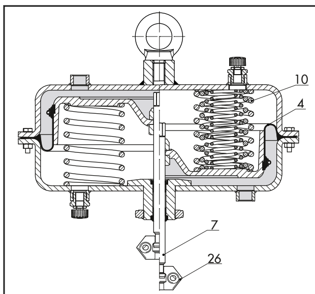
Fig. 2: Typ 3271, 1400-60 cm 2 · Rörelseriktning "Ställdonets spindel dras in" (vänster) · Extra fjädrar och rörelseriktning "ställdonets spindel skjuts ut" (höger)
