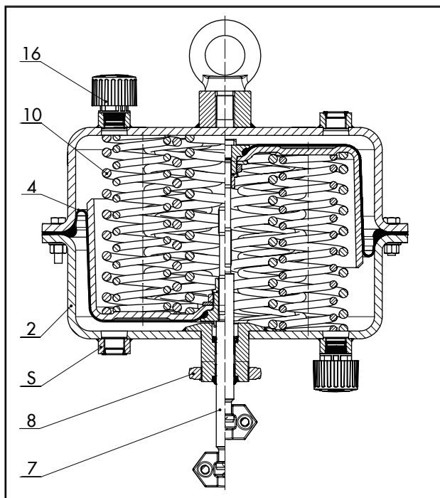
Fig. 2: Typ 3271 med 1000 cm 2 ställdonsområde
