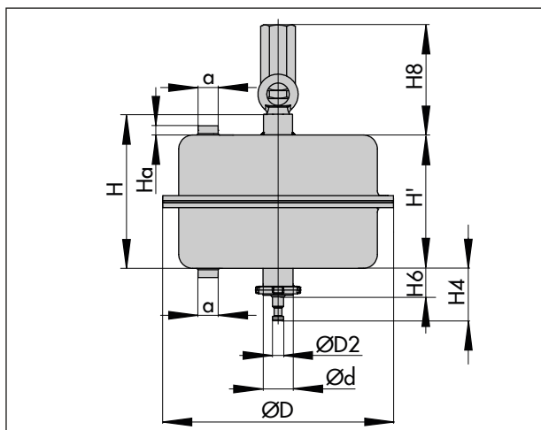
Fig. 4: 1000 cm 2 ställdonsområde, med justerbart slaglängdsstopp
