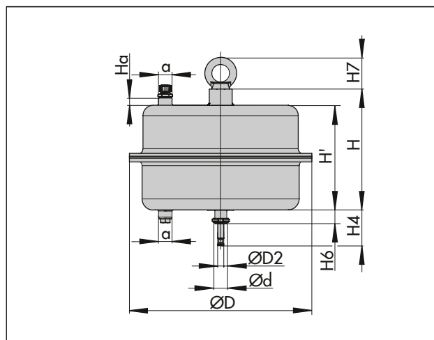
Fig. 3: Typ 3271 med 1000 cm 2 ställdonsområde
