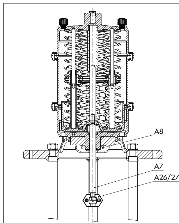
Afbeelding 7: Pneumatische aandrijving typ 3271 wordt op de slagventiel aangebouwd
