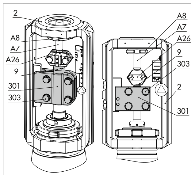
Afbeelding 8: Zekering tegen verdraaien: standaarduitrusting in afbeelding links, afwijkende uitvoering in het figuur rechts
