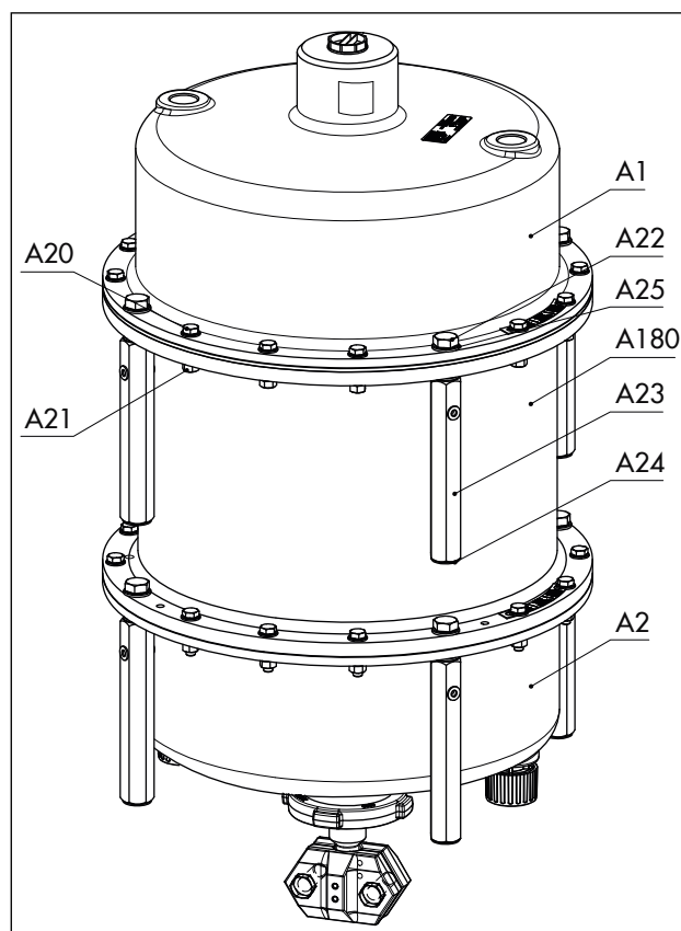
Afbeelding 9: Aandrijving met spanschroeven en spanmoeren
