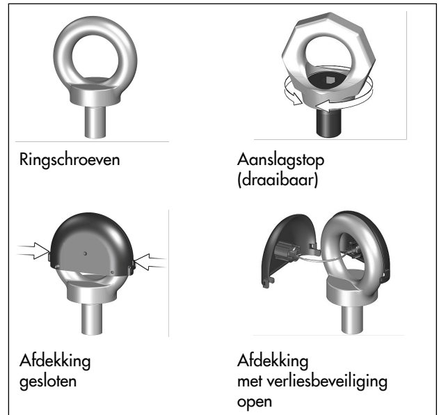
Afbeelding 4: Verliesbeveiliging aan ringschroeven/aanslagstop
