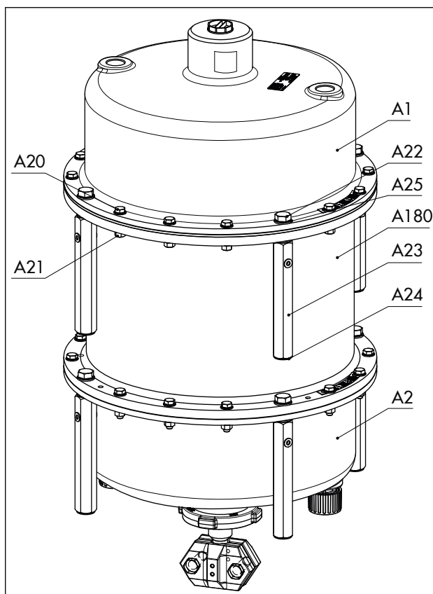
Afbeelding 10: Aandrijving met spanschroeven en spanmoeren
