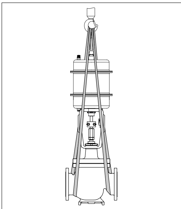
Afbeelding 6: Hefpunten op het regelventiel (voorbeeld)
