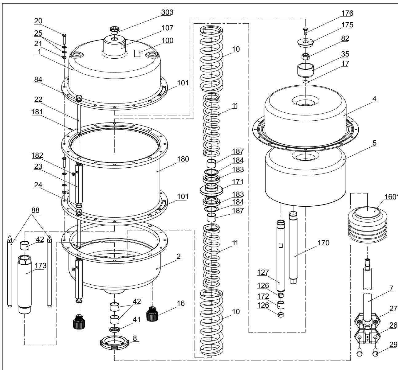
Afbeelding 11: Aandrijving van het type 3271, 1400-250 cm 2
