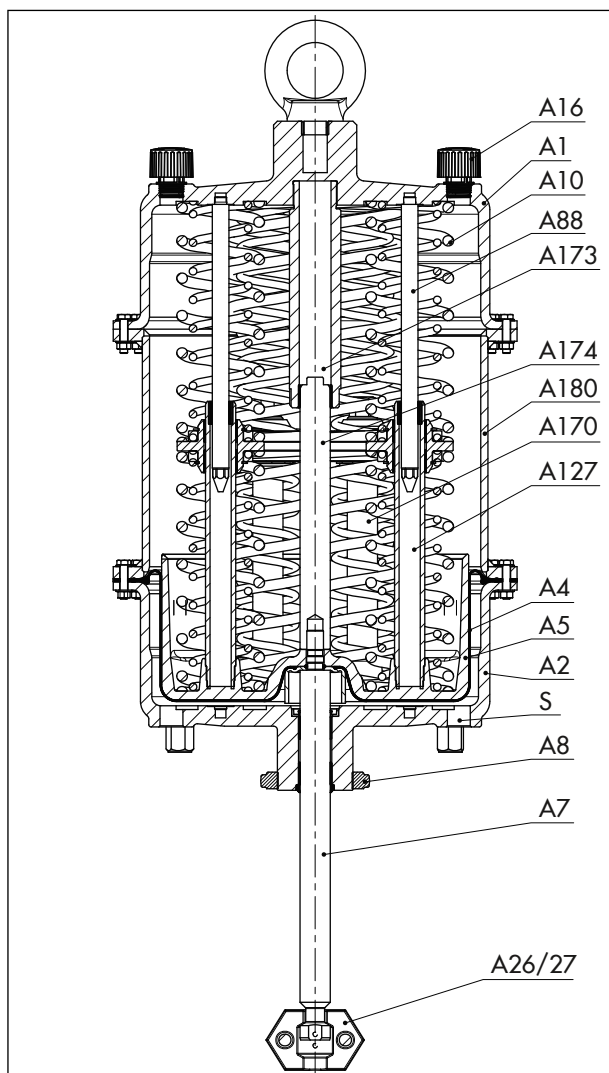
Afbeelding 2: Pneumatische aandrijving van het type 3271, voorbeeldafbeelding met een aandrijvingsoppervlak van 1400-250 \text{ cm}^2
