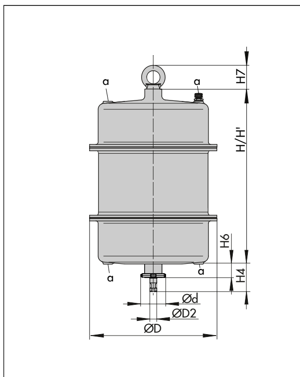
Afbeelding 3: Type 3271 met een aandrijvingsoppervlak van 1400-250 cm 2
