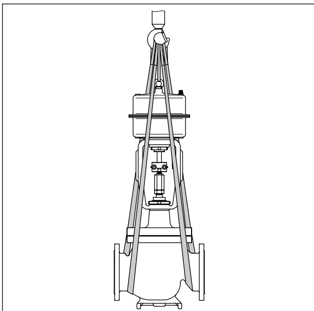
Afbeelding 9: Hefpunten op het regelventiel (voorbeeld)
