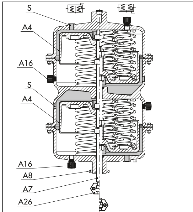
Afbeelding 3: Pneumatische aandrijving van het type 3271, voorbeeldafbeelding met 2x een aandrijvingsoppervlak van 2800 cm 2
