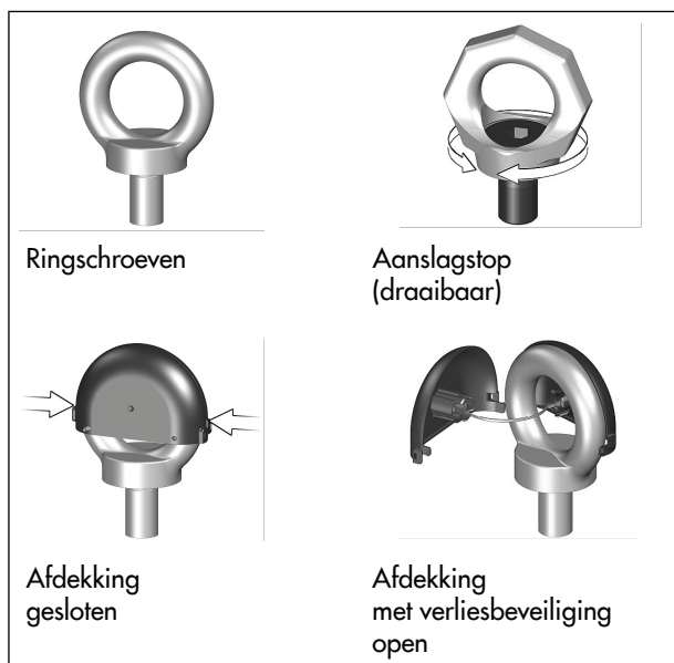
Afbeelding 7: Verliesbeveiliging aan ringschroeven/aanslagstop
