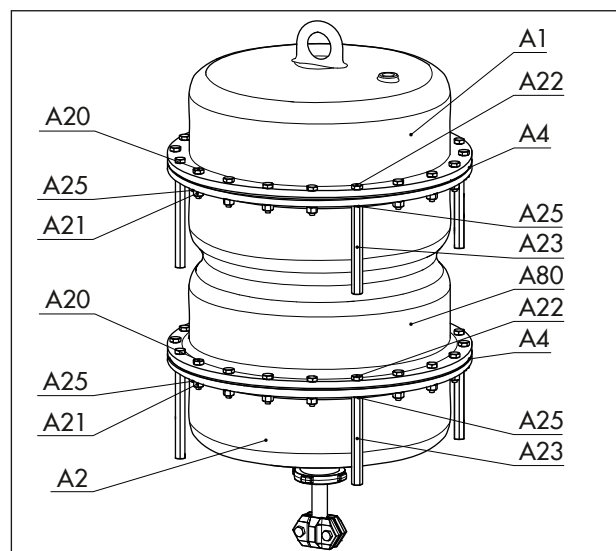
Afbeelding 13: Tandemaandrijving met spanschroeven en spanmoeren
