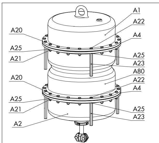
Afbeelding 16: Tandemaandrijving met spanschroeven en spanmoeren
