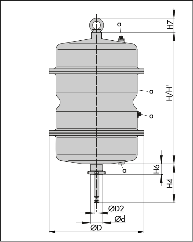
Afbeelding 6: Type 3271 als tandemaandrijving
