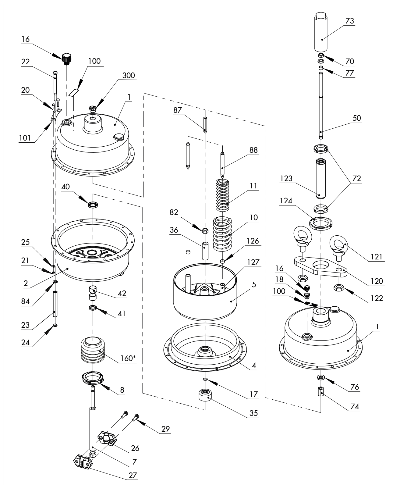
Afbeelding 17: Aandrijving van het type 3271, 1400-120 cm 2
