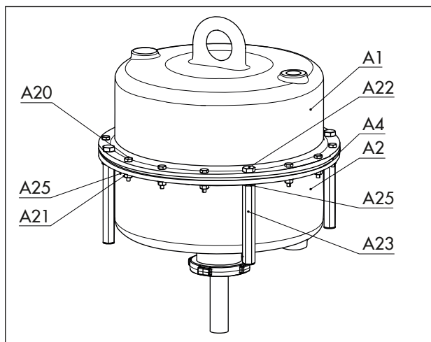
Afbeelding 15: Aandrijving met spanschroeven en spanmoeren
