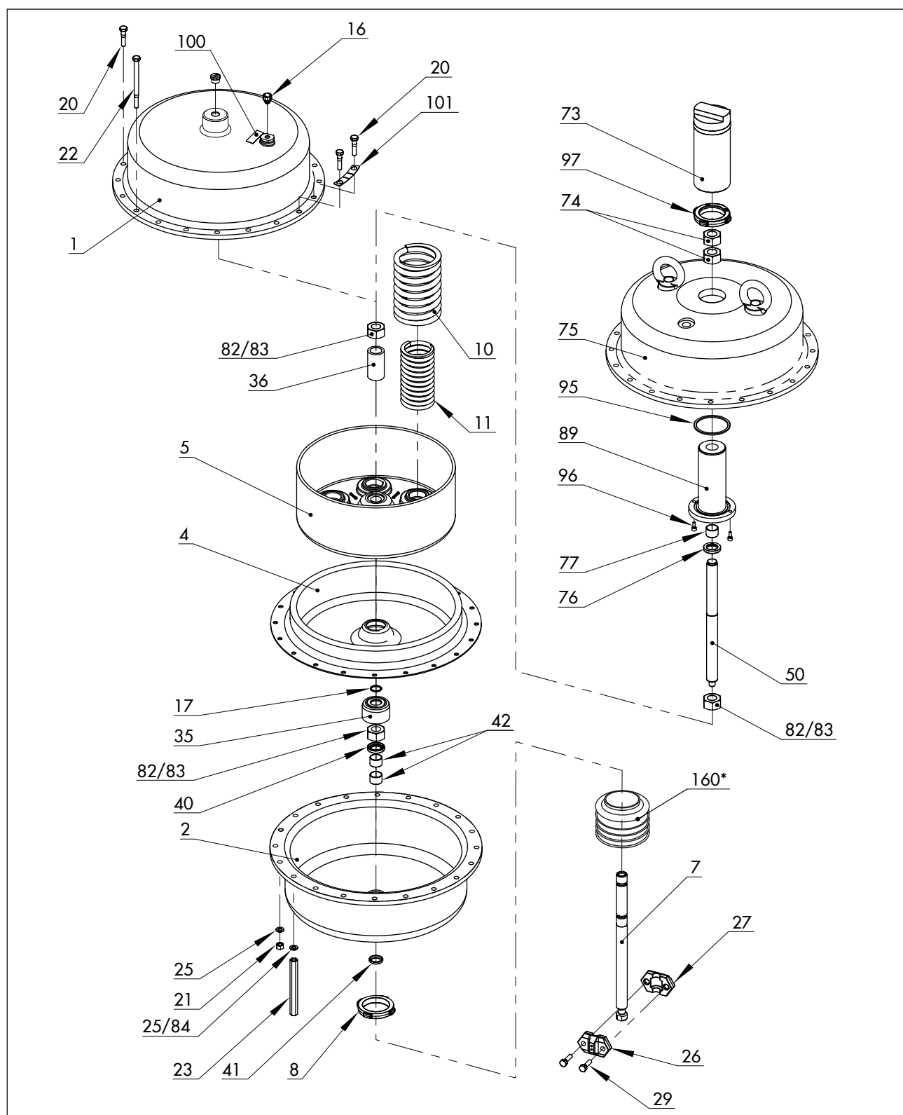
Afbeelding 18: Aandrijving van het type 3271, 2800 cm 2
