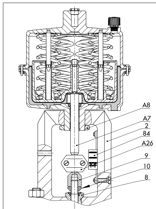
Afbeelding 10: Pneumatische aandrijving typ 3271 wordt op de slagventiel aangebouwd
