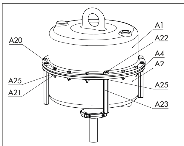
Afbeelding 12: Aandrijving met spanschroeven en spanmoeren
