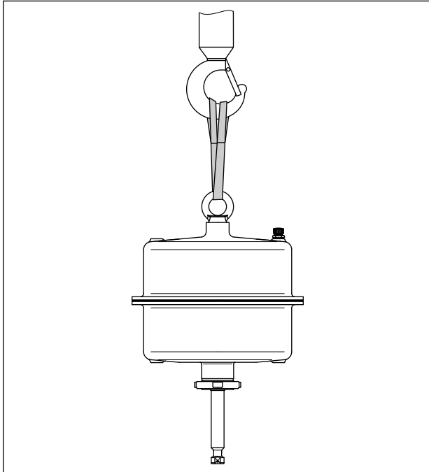
Afbeelding 8: Hefpunt op de aandrijving
