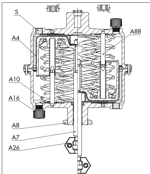
Afbeelding 2: Pneumatische aandrijving van het type 3271, voorbeeldafbeelding met een aandrijvingsoppervlak van 1400-120 \text{ cm}^2
