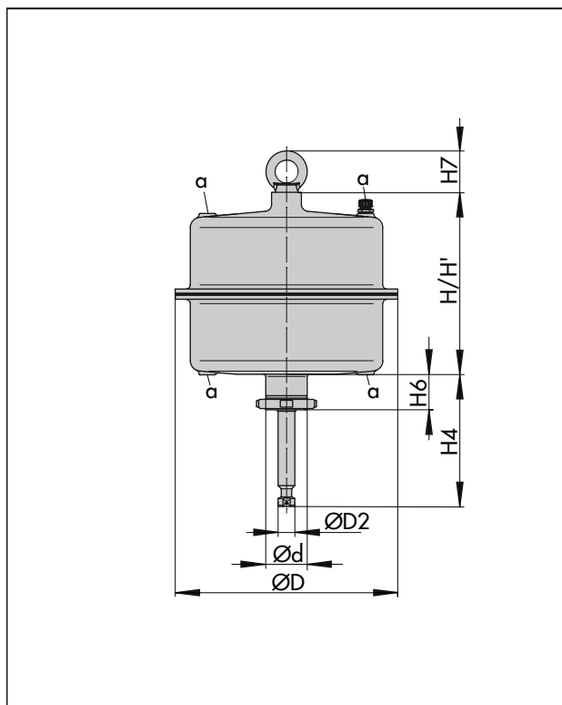
Afbeelding 4: Type 3271 met een aandrijvingsoppervlak van 1400-120 cm 2
