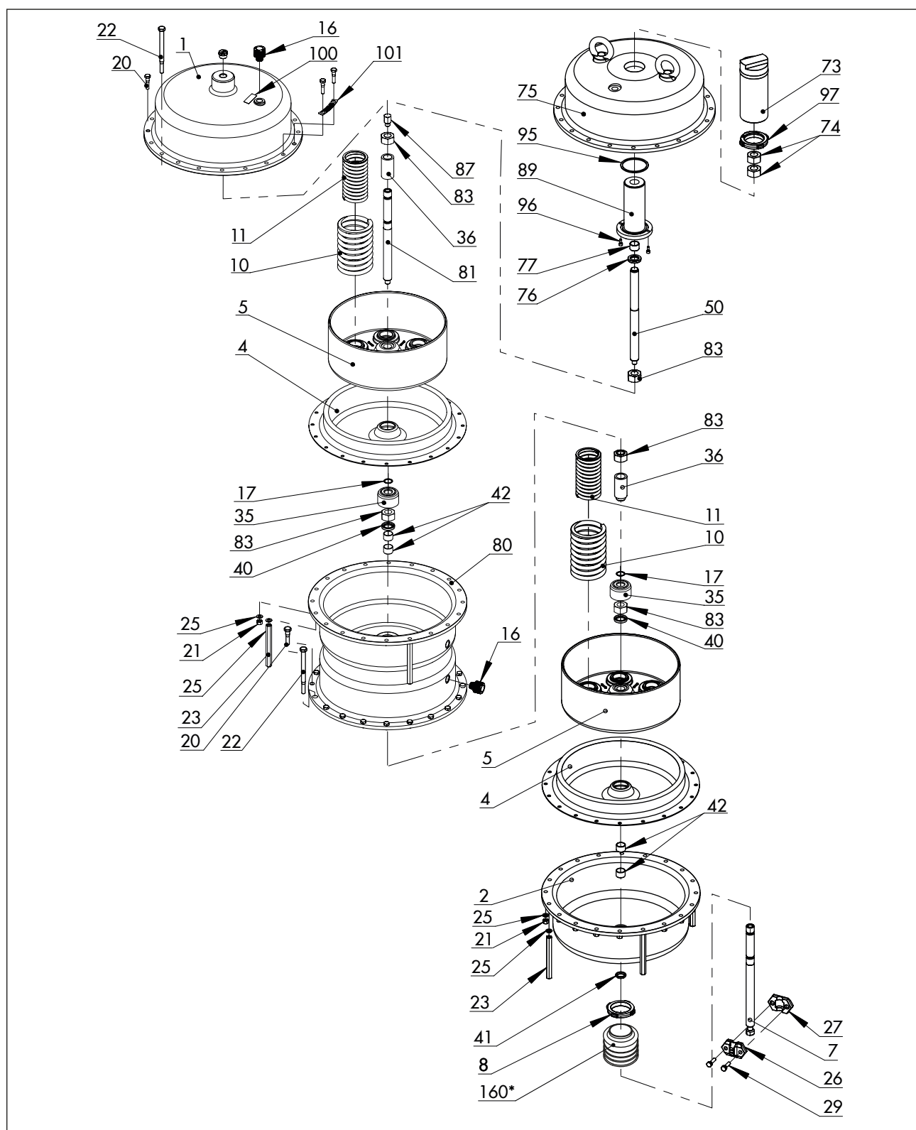
Afbeelding 19: Aandrijving van het type 3271, 2x 2800 cm 2
