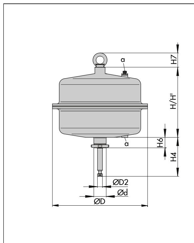
Afbeelding 5: Type 3271 met een aandrijvingsoppervlak van 2800 cm 2
