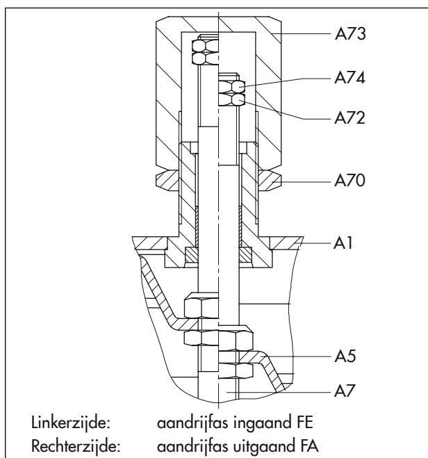
Afbeelding 14: Slagbegrenzing
