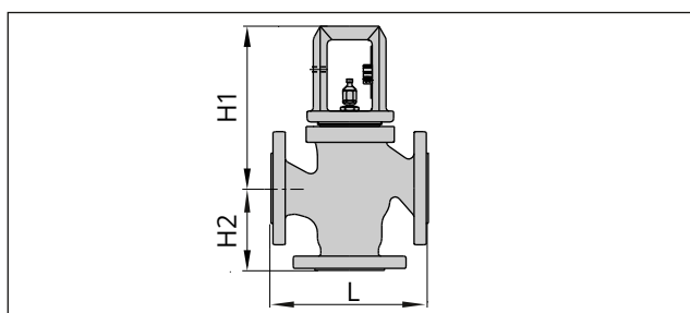
Fig. 6 : Vanne type 3244
