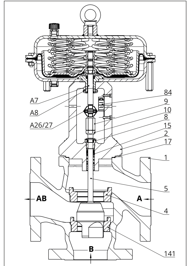
Fig. 4 : Vanne type 3244 en vanne de mélange avec servomoteur pneumatique type 3271
