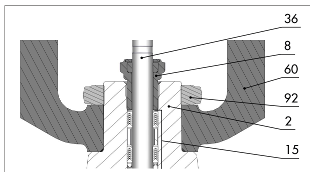
Fig. 11 : Garniture avec presse-étoupe vissé au centre (exemple)
