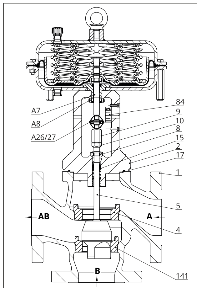
Fig. 13 : Vanne type 3244 en vanne de mélange avec servomoteur pneumatique type 3271
