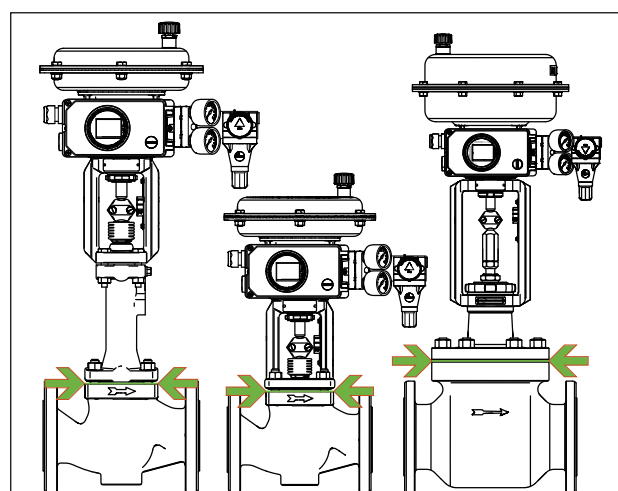
Fig. 9 : Limite d'isolation des vannes de régulation (exemple)
