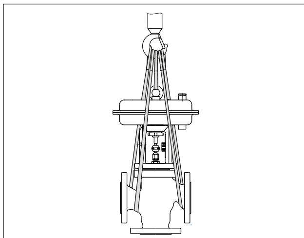
Fig. 8 : Points de levage sur la vanne de régulation
