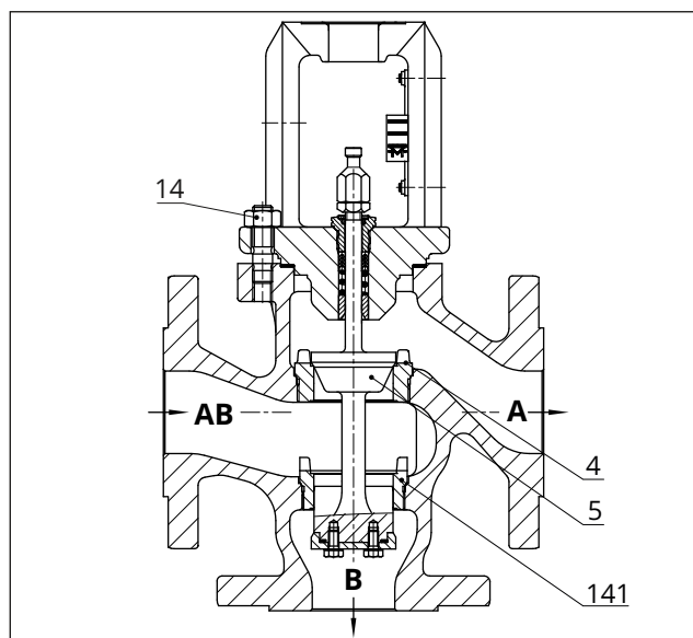
Fig. 5 : Vanne type 3244 en vanne de répartition
