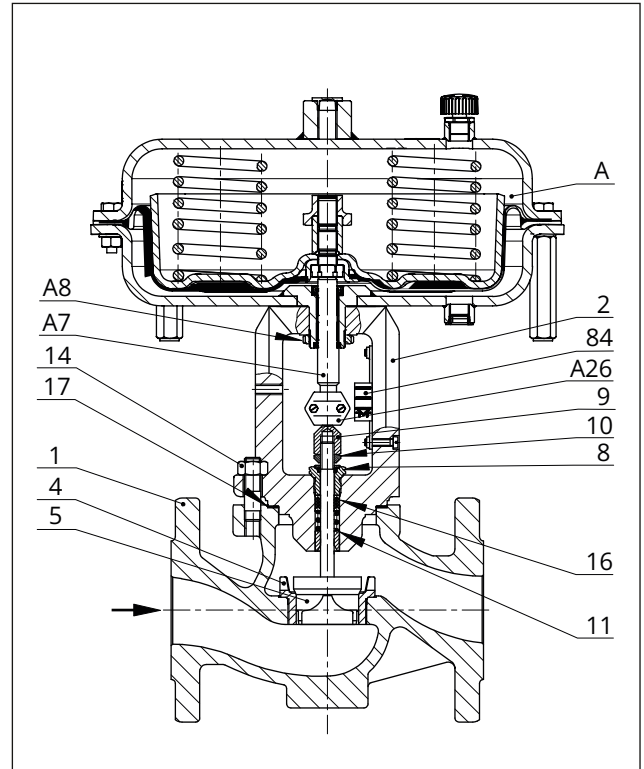
Fig. 24: Valvola di regolazione Tipo 3241-1 con attuatore pneumatico Tipo 3271, alloggiamento fino a DN 150/NPS 6
