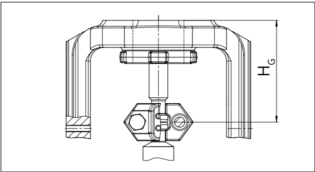
Fig. 21: Misura di riferimento accoppiamento/castello
