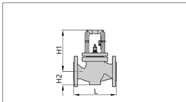
Fig. 13: Tipo 3241 fino a diametro nominale DN 150/NPS 6/ DN 150A
