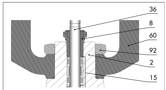
Fig. 22: Avvitare centralmente il pacco con la boccola filettata (esempio)
