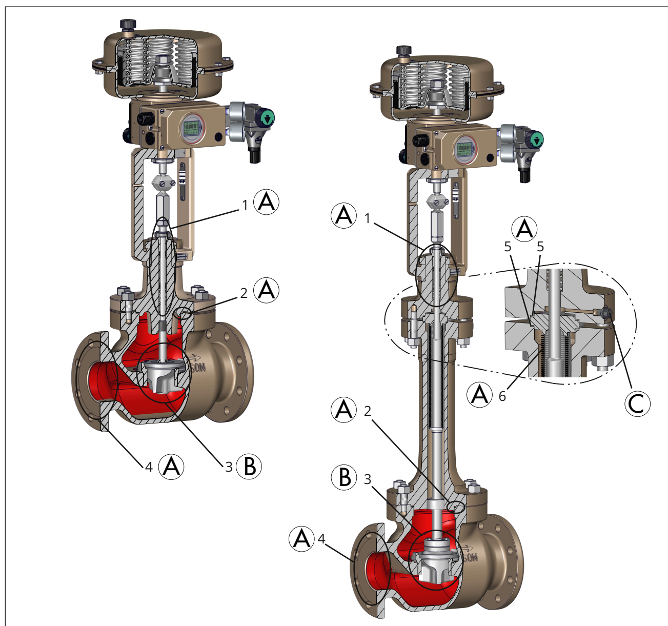
Fig. 23: Possibili punti di perdita nella valvola di controllo (esempi: a sinistra versione con parte superiore standard, a destra versione con soffietto, rappresentativa anche delle versioni con parte isolante o adattatore).
