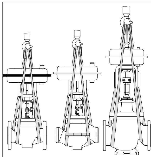
Fig. 14: Punti di sollevamento sulla valvola di regolazione: fino a DN 150/NPS 6 con flange (sinistra) e con estremità saldate (centro) · a partire da DN 150/NPS 6 con occhiello di sollevamento aggiuntivo sull'attuatore (destra)
