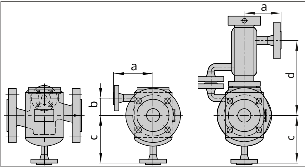
Fig. 11: Tipo 3241 con mantello di riscaldamento fino a diametro nominale DN 100/NPS 4 · nella figura a destra con parte isolante o a soffietto
