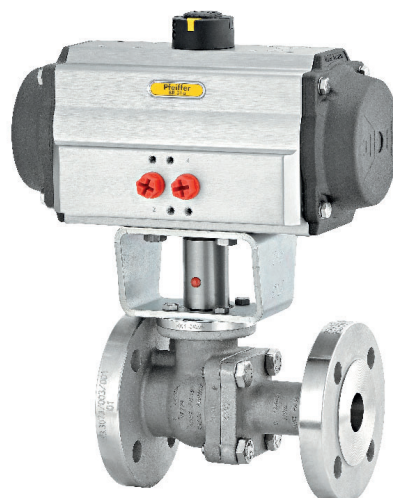
Figure 2: Vanne à boisseau sphérique BR 26d avec servomoteur rotatif BR 31a
